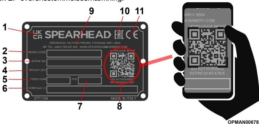
Figur 2 – Serienummerplade
