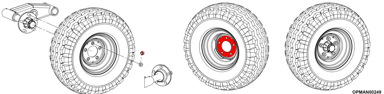
Figur 5.73 – Retning for hjul og hjulmøtrik på Stubble Master
