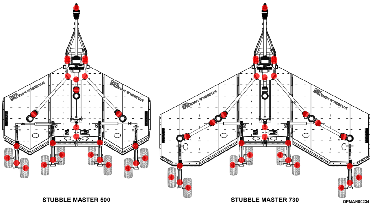
Figur 5.8 – Placeringer af smørepunkter på Stubble Master
