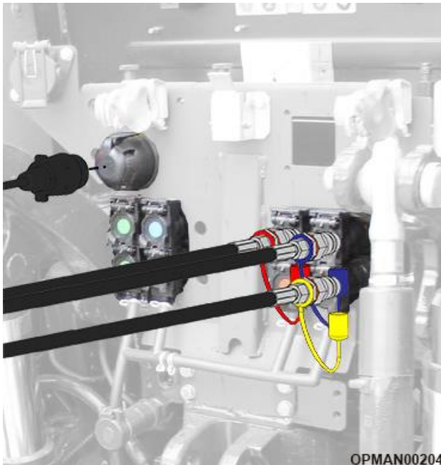
Figur 4.3 Slange- og lygtetilslutninger på Stubble Master
