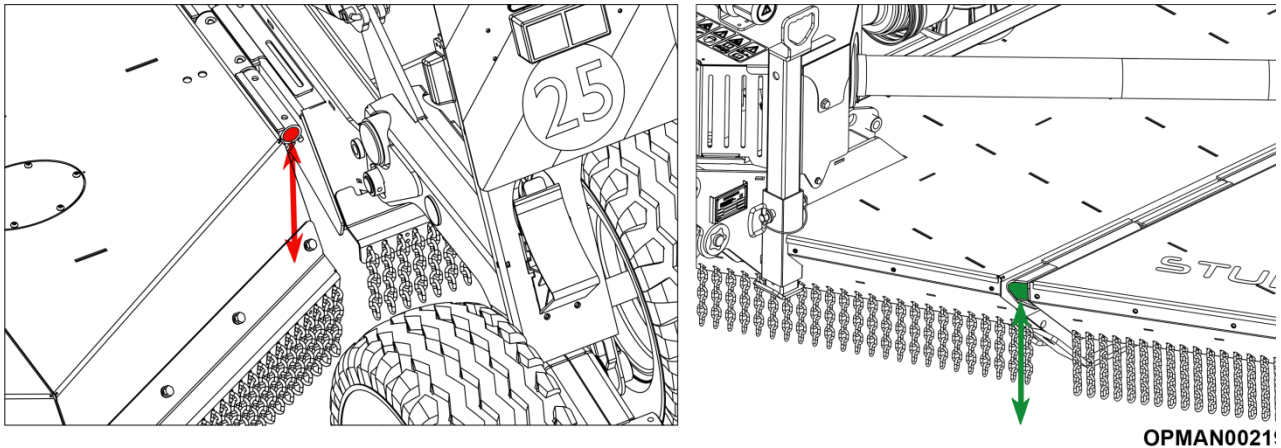
Figur 4.19 – Nivellering af Stubble Master 500/730-maskine fra forrest til bagest (Stubble Master 500-model vist)
