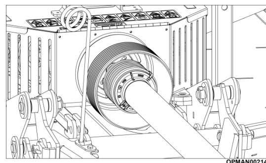
Figur 4.13 – Monter på Stubble Master
