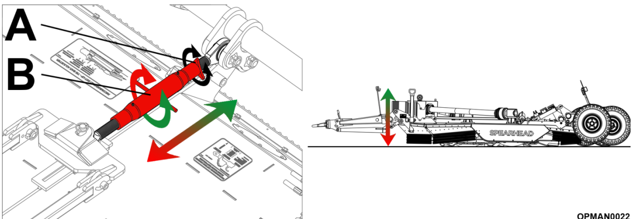
Figur 4.20 – Nivellering af Stubble Master 500/730-maskine fra forrest til bagest (Stubble Master 500-model vist)
