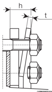
Figur 5.46 – Vejledning til dimensioner for koblingsindstilling
