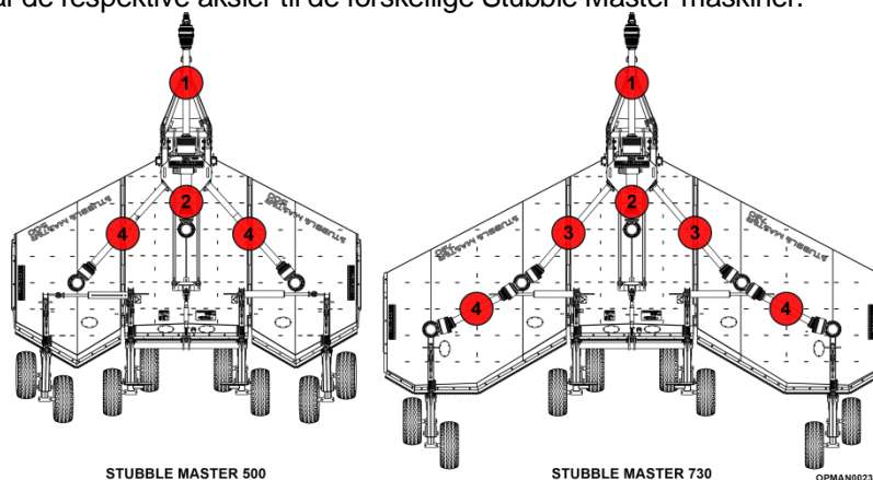
Figur 5.4 – Placeringer af indgangsaksletyper på Stubble Master
