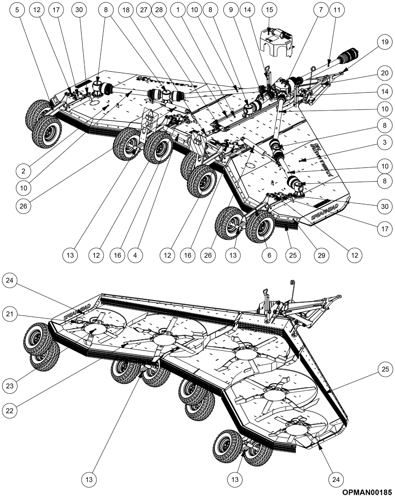
Figur 1.3 – Generel opsætning for Stubble Master 730
