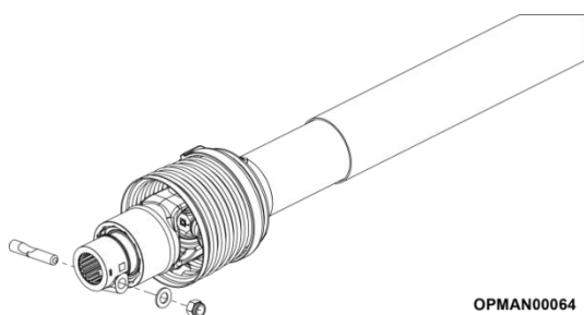
Figur 4.12 – Fjern konisk stift
