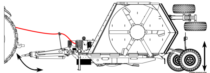
Figur 4.7 – Højdejustering af trækøje
