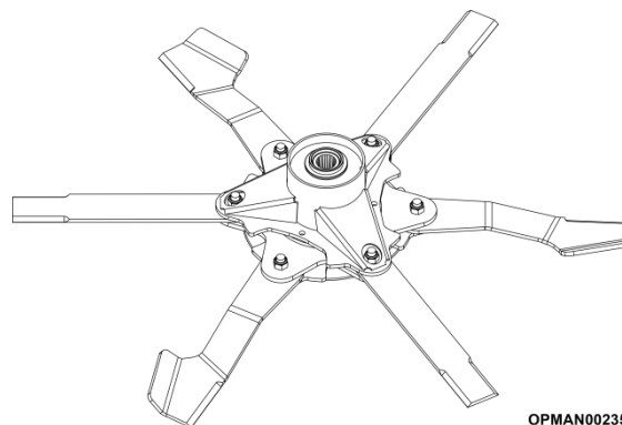
Figur 5.47 – Knivenhed på Stubble Master
