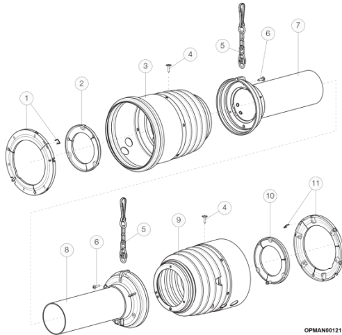
Figur 5.9/tabel 5.8 – Sikkerheds- og slidkomponenter til indgangsaksel
