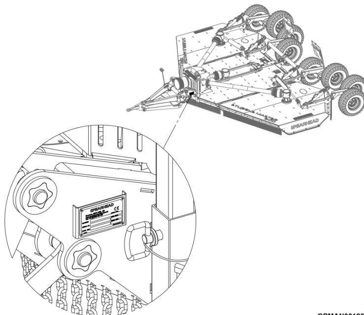
Figur 1.5 – Placering af serienummerplade (500-model illustreret)
