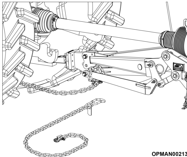
Figur 4.10 – Sikkerhedskæde til bugsering
