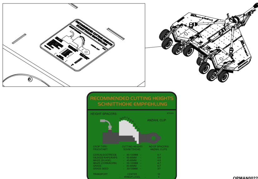
Figur 4.26 – Mærkat med anbefalet klippehøjde på midterskjold og placering
