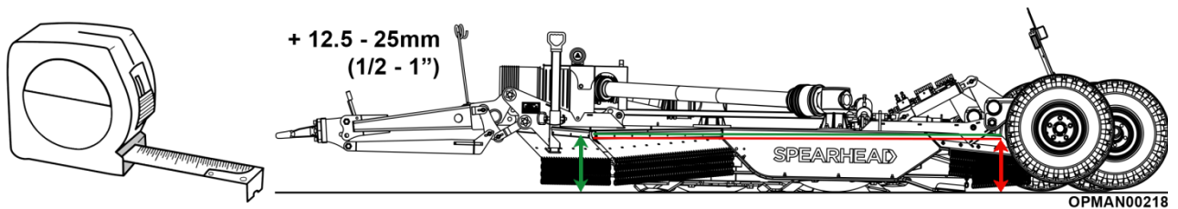
Figur 4.18 – Nivellering af Stubble Master 500/730-maskine fra forrest til bagest (Stubble Master 500-model vist)
