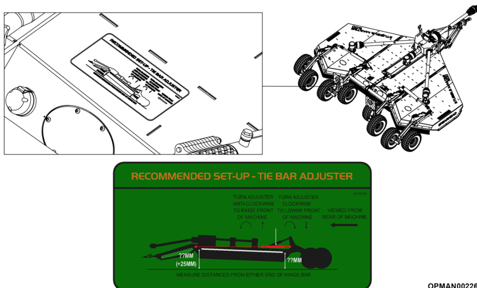
Figur 4.22 – Mærkat for justering af midterskjoldets fastgørelsesstang og placering
