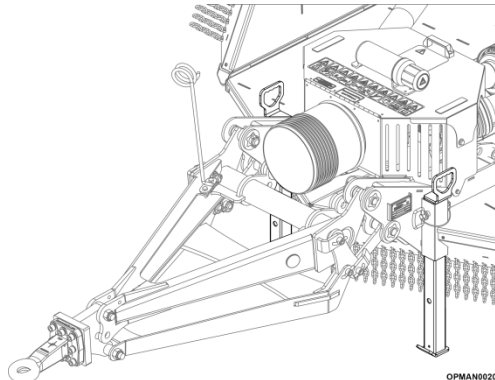
Figur 3.3 – Placering af stativ på Stubble Master
