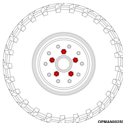
Figur 5.74 – Hjulmøtrikker, der skal løsnes på gaffeltruckdæk på Stubble Master
