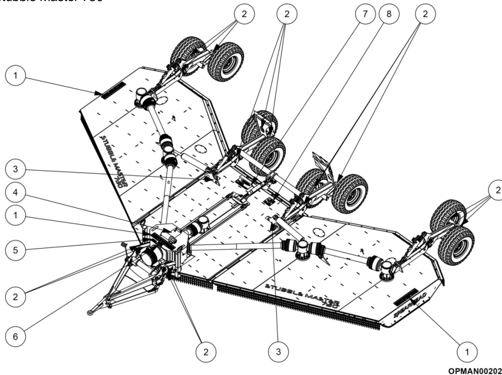
Figur 2.4 – Placering af sikkerheds- og instruktionsmærkater på Stubble Master 730
