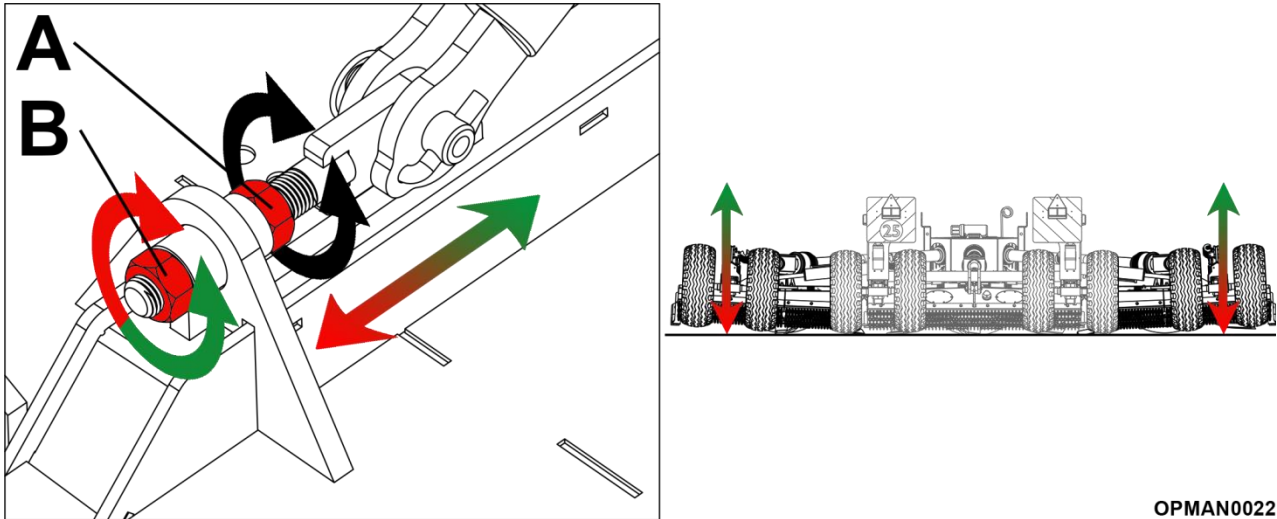
Figur 4.24 – Justering af vingeksel for nivellering af maskine fra venstre til højre
