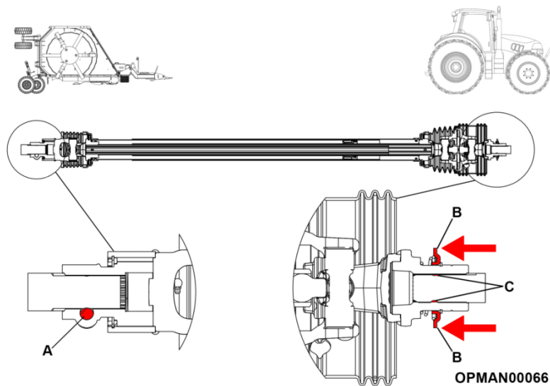
Figur 4.11 – På- og afmontering af indgangsaksel på Stubble Master
