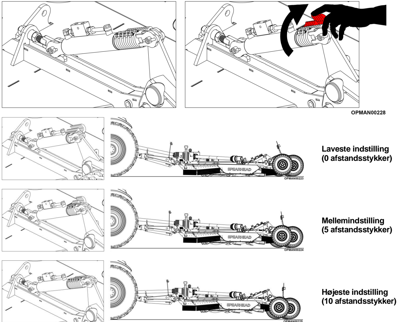
Figur 4.25 – Indstilling af klippehøjde på Stubble Master med afstandsstykker
