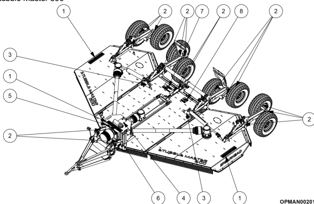
Figur 2.3 – Placering af sikkerheds- og instruktionsmærkater på Stubble Master 500
