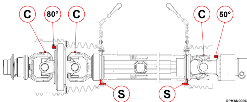
Figur 5.5 – Smørepunkter på Stubble Master-indgangsaksler
