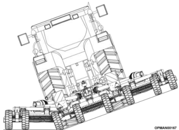
Figur 4.32 – Traktorens stabilitet
