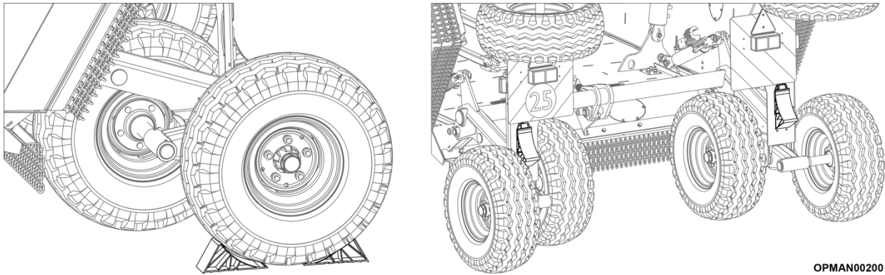
Figur 3.2 – Placering og opbevaring af stopklodser på Stubble Master
