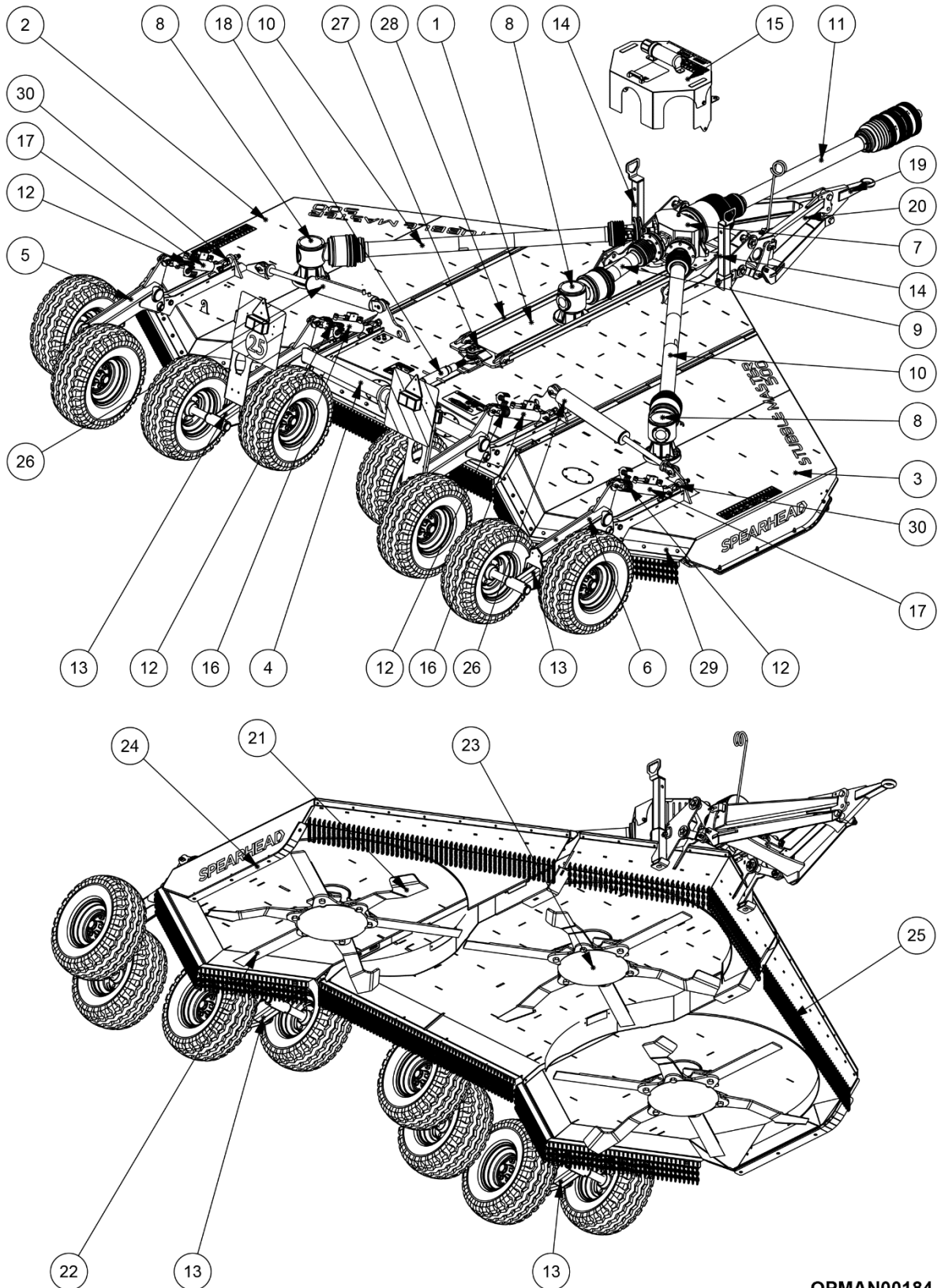
Figur 1.2 – Generel opsætning for Stubble Master 500
