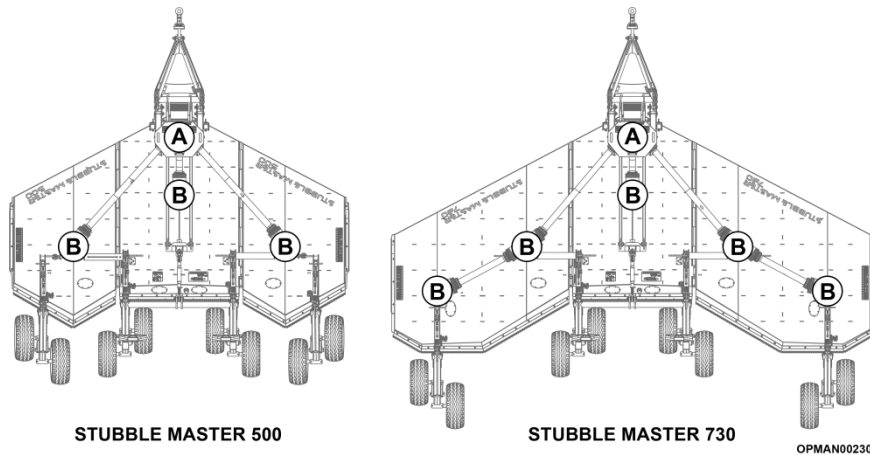
Figur 5.1 – Placeringer – oliekapaciteter i Stubble Master-gearkasse
