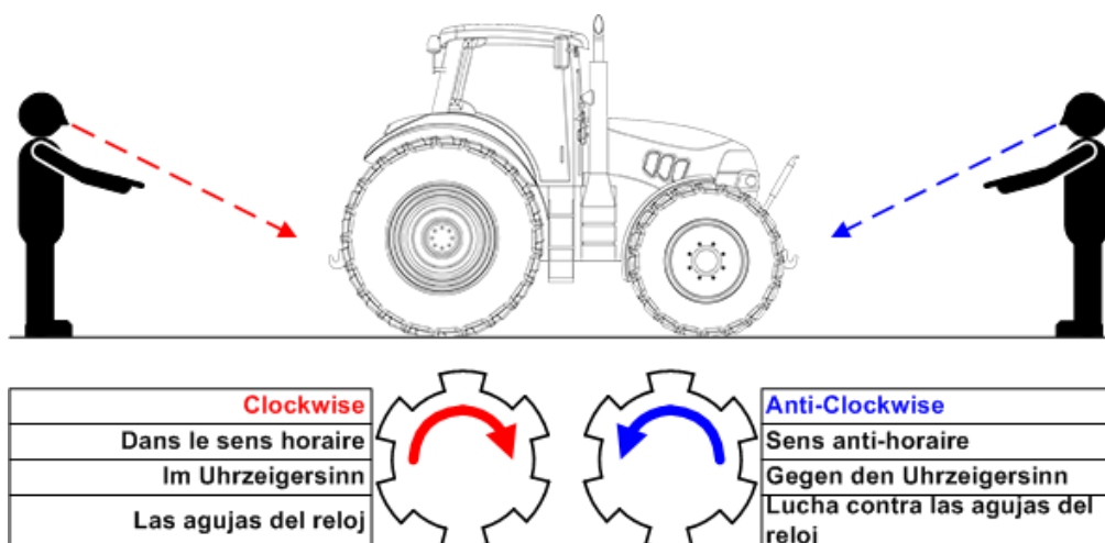
Figur 1.8 – Definitioner af rotation for traktorens PTO-aksel
