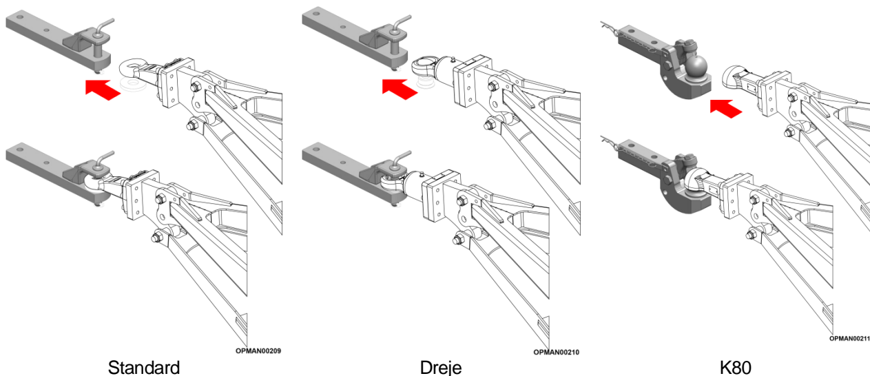
Figur 4.8 – Trækøjemuligheder på Stubble Master
