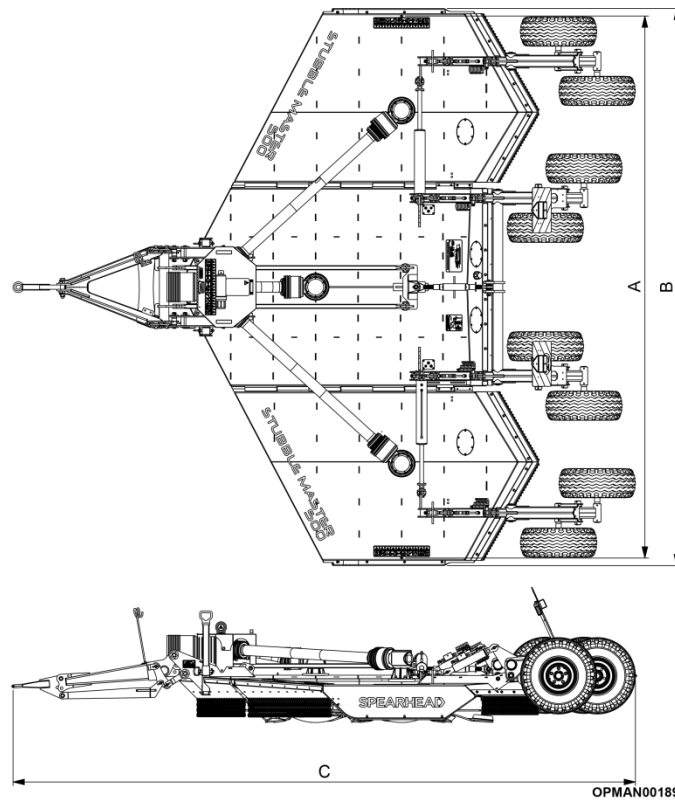
Figur 1.9 Arbejdsdimensioner
