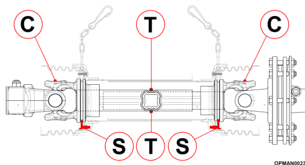
Figur 5.6 – Smørepunkt på Stubble Master-centeraksel
