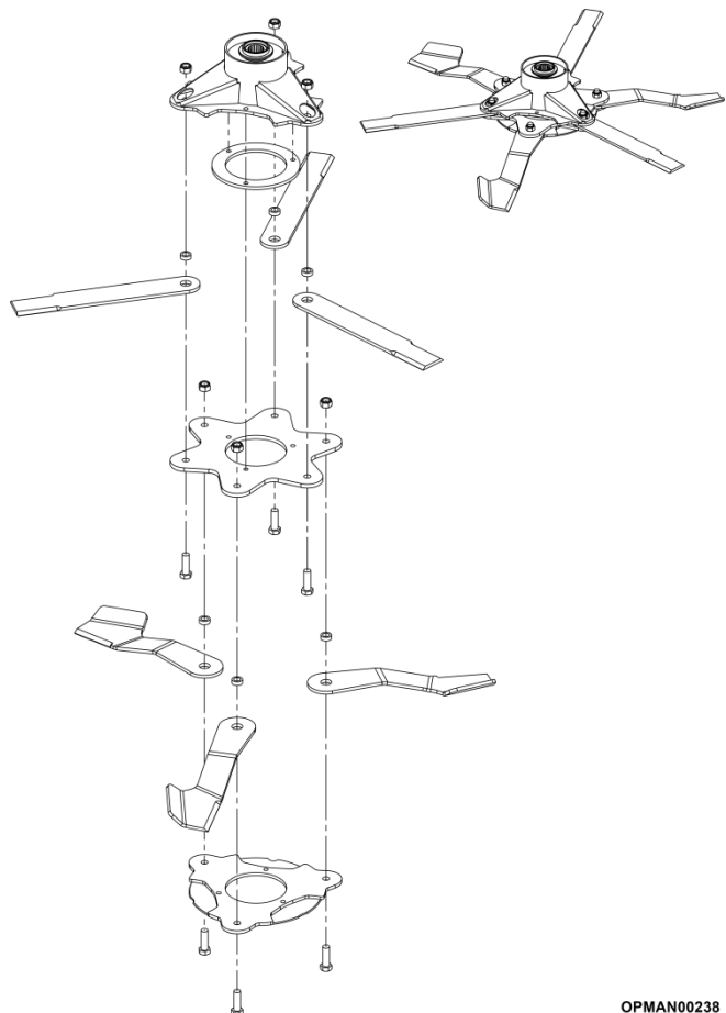
Figur 5.48 – Knivholderenhet på Stubble Master
